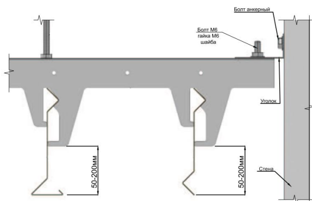
Узел А
