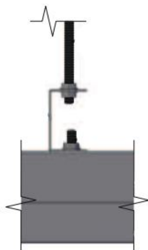
Узел 1
