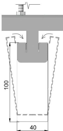
Узел А
