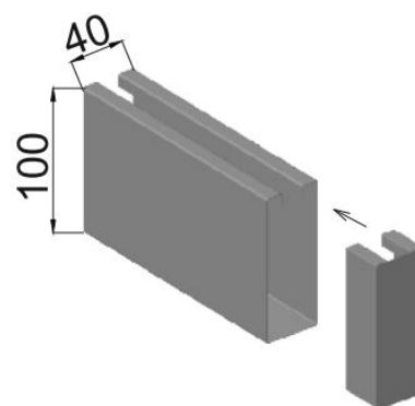
Узел Б
