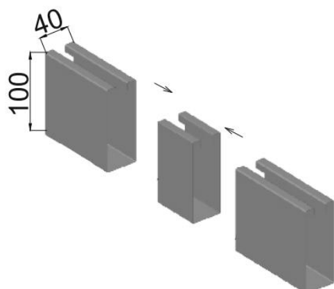
Узел А
