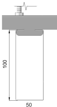
Узел А
